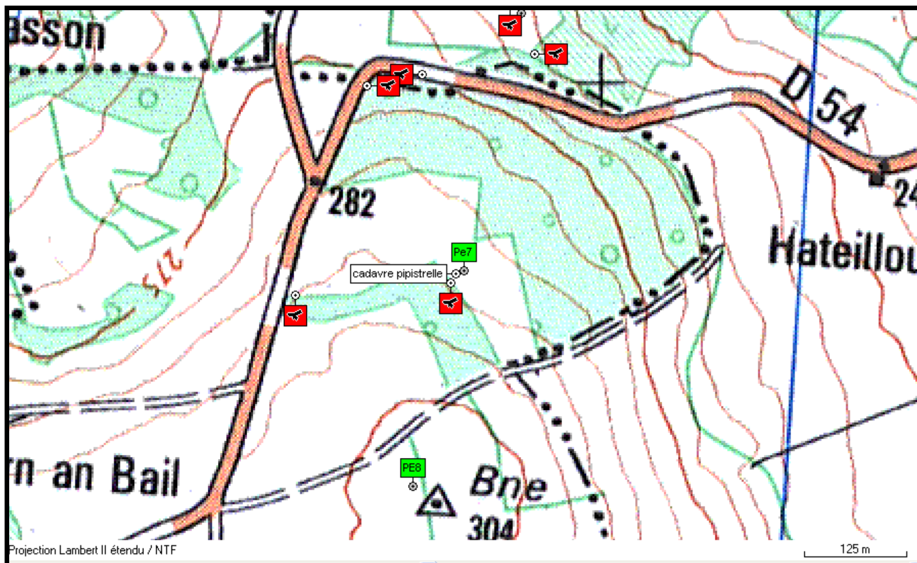
Carte n° 8 : contacts et mortalité de Pipistrelle commune .
