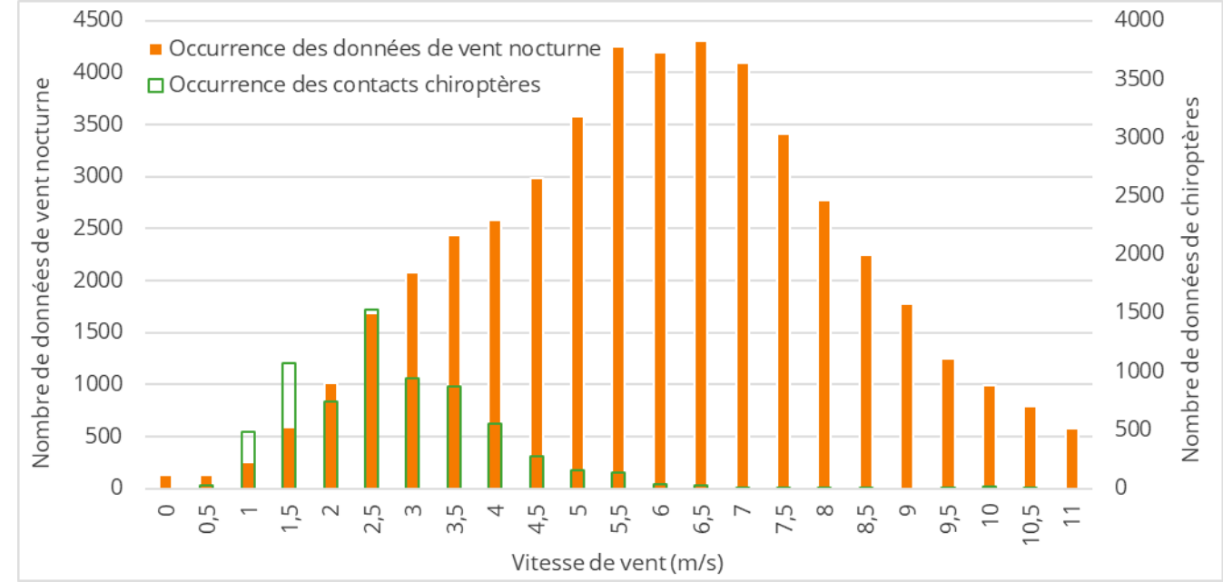
Figure 26 : Activité des chiroptères en fonction de la vitesse du vent
