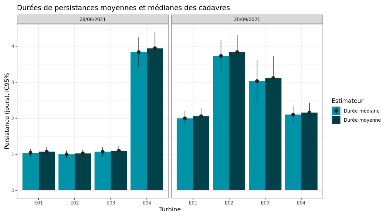
Figure 20 : Durées de persistance moyennes accompagnées des incertitudes (intervalles de confiance à 95%) des cadavres pour chaque test de prédation (28 juin et 20 septembre 2021)
