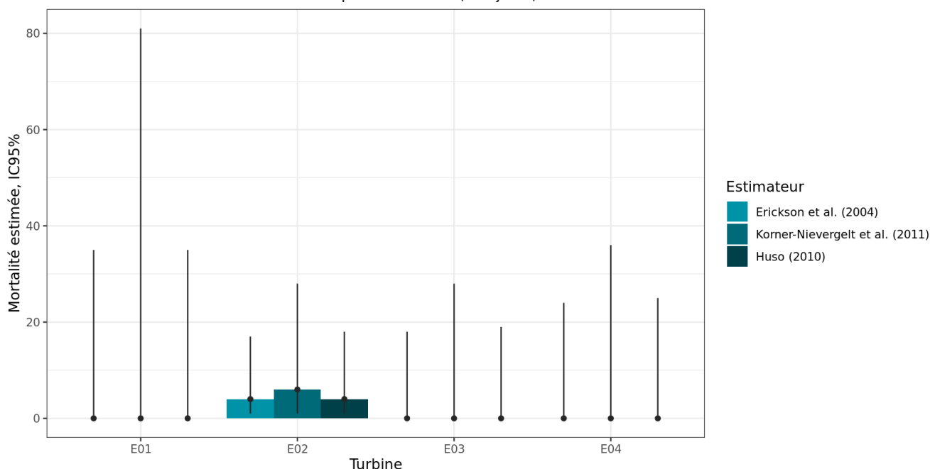
Figure 22 : Estimation de la mortalité la plus probable (et incertitude à 95%) pour les oiseaux pour le parc éolien de Cast 2 au cours du suivi de 2021 sur 160 jours.
