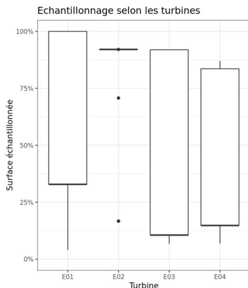
Figure 12 : Bilan des surfaces prospectées par éolienne sur l'ensemble du suivi. Synthèse (boîte à moustaches) du pourcentage de surface prospectée par passage par éolienne sur l'ensemble du suivi (de bas en haut : minimum, 1er quartile, médiane en gras, 3ème quartile, maximum).
