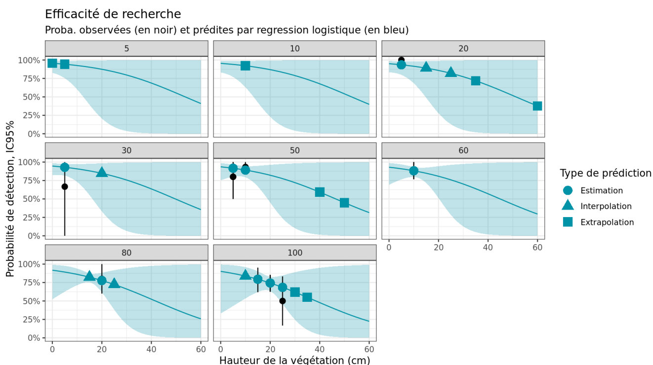
Figure 21 : Efficacité de recherche et probabilité de détection des cadavres selon la hauteur et le recouvrement
