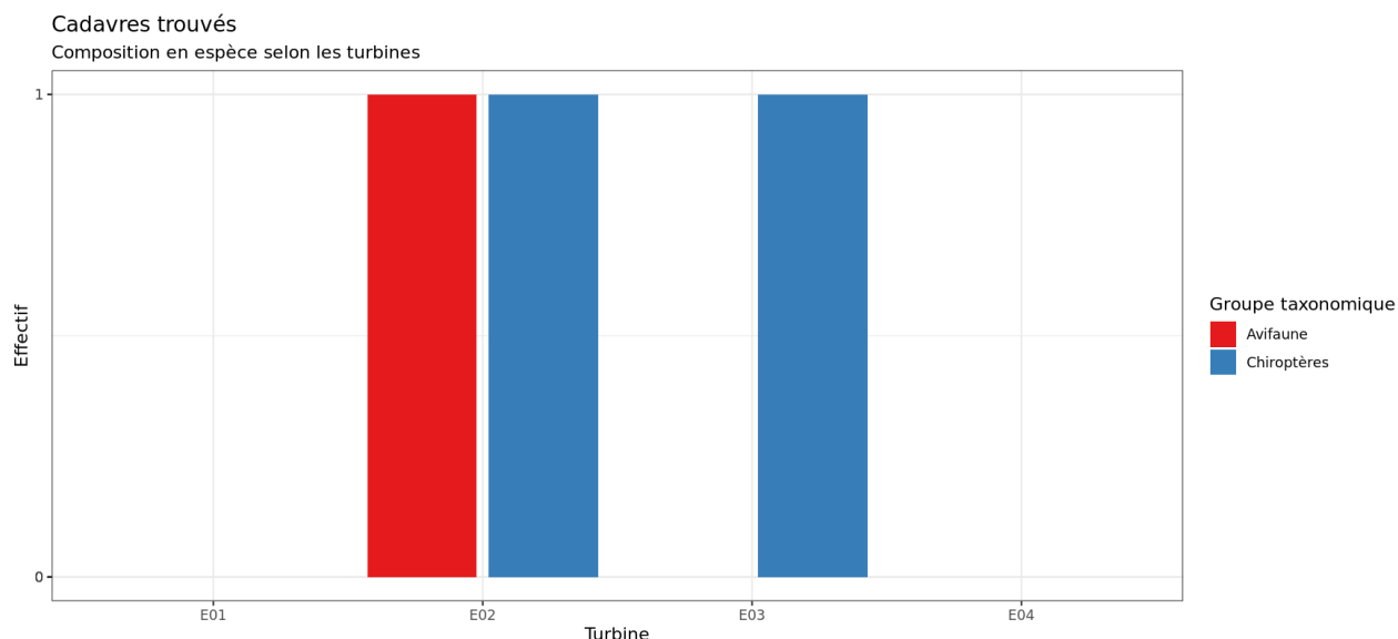
Figure 17 : Nombre de cadavres découverts par éolienne
