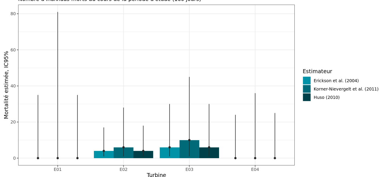
Figure 23 : Estimation de la mortalité la plus probable (et incertitude à 95%) pour les chiroptères pour le parc éolien de Cast 2 au cours du suivi de 2021 sur 160 jours
