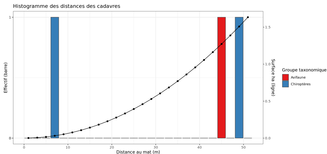
Figure 18 : Répartition spatiale (distance à l'éolienne) des cadavres retrouvés au sein du parc de Cast 2. La courbe représente l'évolution de la surface de l'aire d'étude prospectée en fonction de la distance au pied de l'éolienne.
