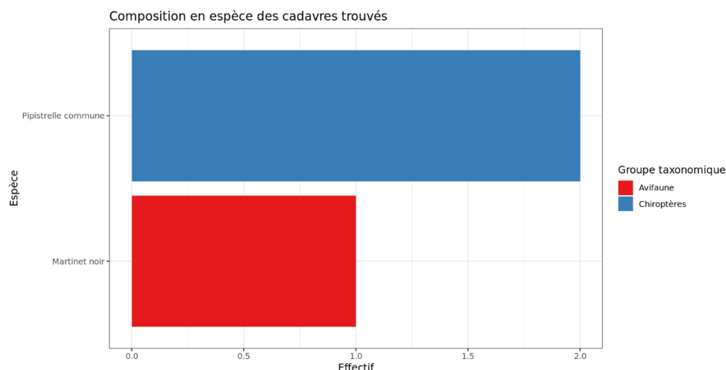
Figure 14 Mortalité par espèce ou groupe d'espèces observée sur le parc éolien de Cast 2
