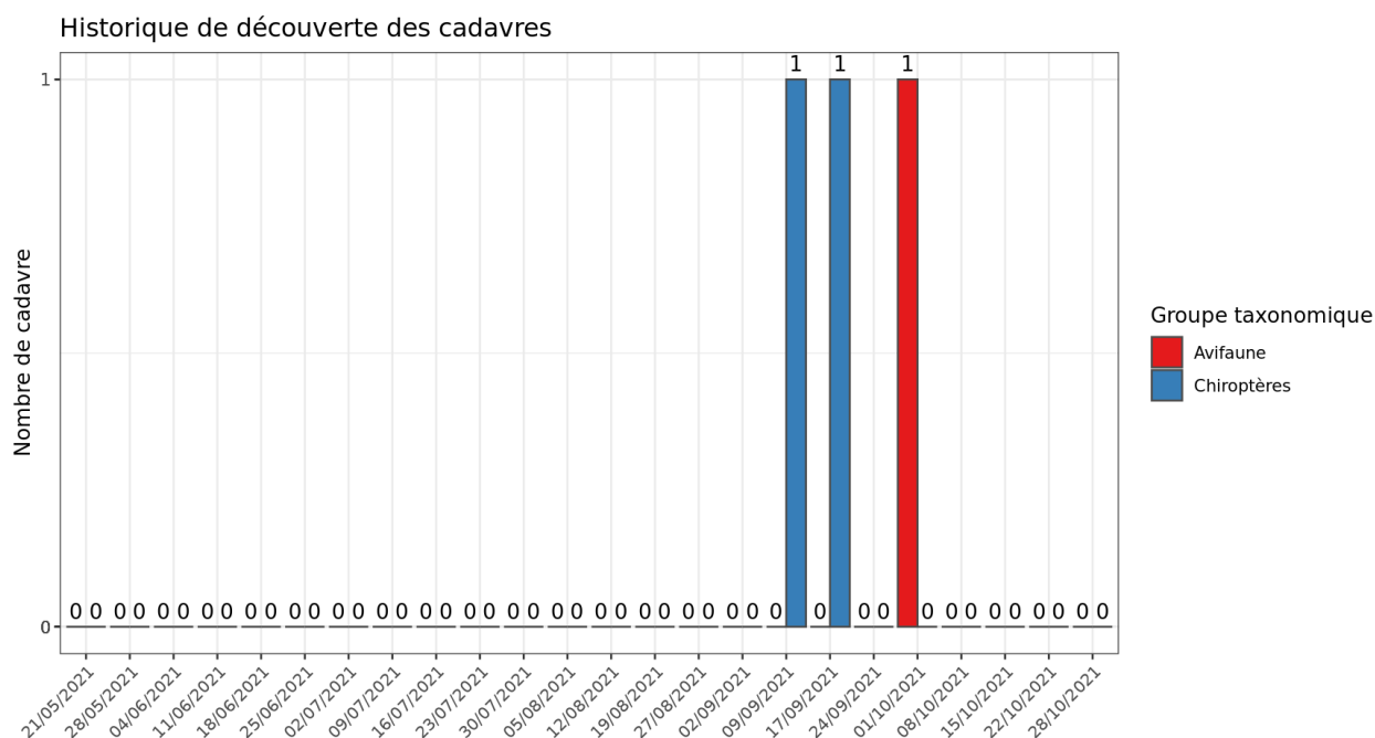
Figure 24 : Phénologie de découverte des cadavres de chiroptères à l'échelle du parc de Cast 2
