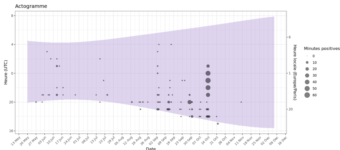
Figure 27 : Actogramme de la Pipistrelle commune pour E02 sur la période du suivi de mortalité
