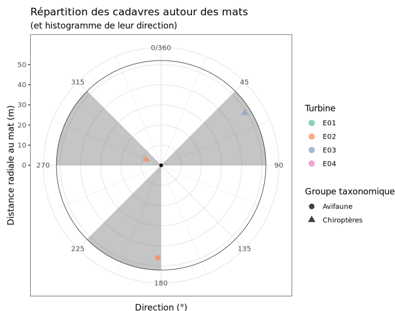
Figure 19 : Positionnement des observations par rapport au positionnement des éoliennes. En grisé, le cumul des observations en histogramme radial en fonction de l'orientation
